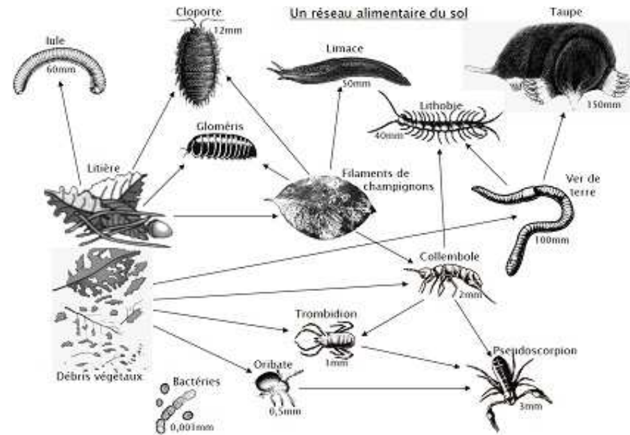
Schéma d'un réseau trophique présent à la surface du sol.
