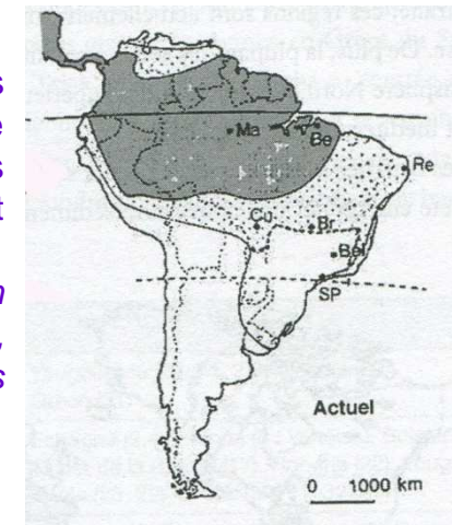
Fig.3 Positions des latérites en Amérique du Sud. En grisé : bauxite; en pointillé : latosols rouges. (D'après Y. Tardy et C. Roquin, ibid ). Les sols latéritiques sont en général des sols peu fertiles, car lessivés de tous leurs nutriments.
